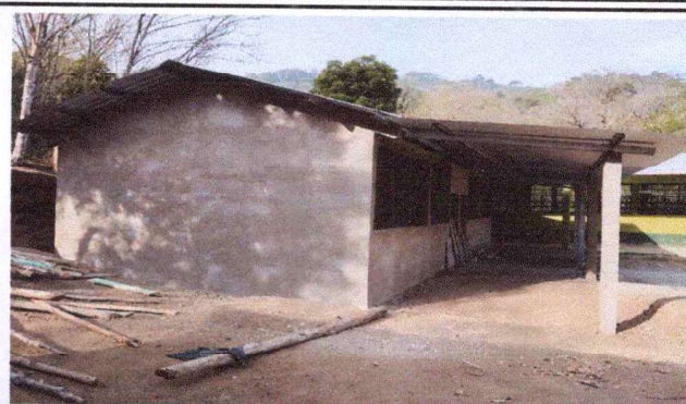
Foto 2: Vista colateral despues de la culminacion de la construccion del proyecto de remozamiento de dos aulas.
